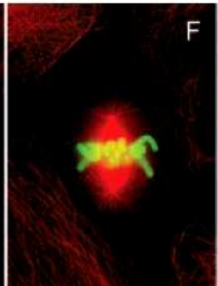
METAPHASE
