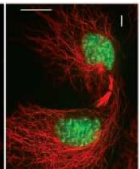
CYTODIERESE
